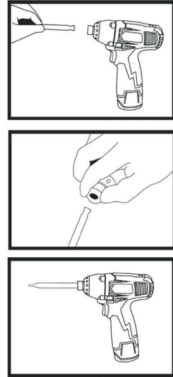
Fig. 3 – Instalación del Bits
