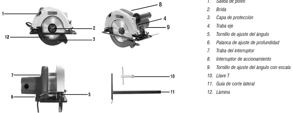
Fig. 2 – Componentes modelo SCD 1400
