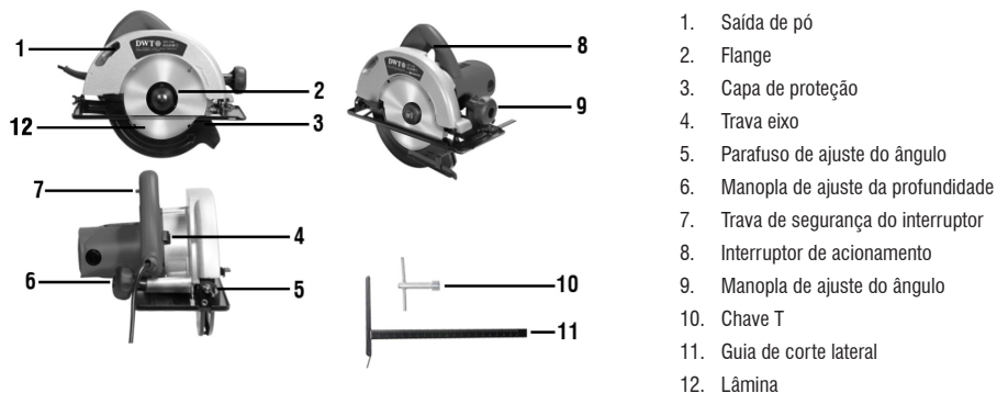
Fig. 1 – Componentes modelo SCD 1100
