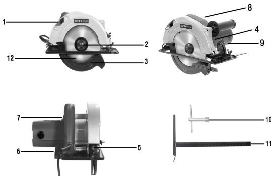
Fig. 2 – Componentes modelo SCD 1400
