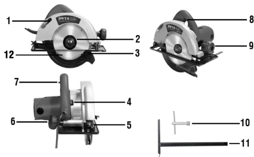
Fig. 1 – Componentes modelo SCD 1100
