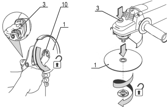
Figura 7 – Substitución del disco
