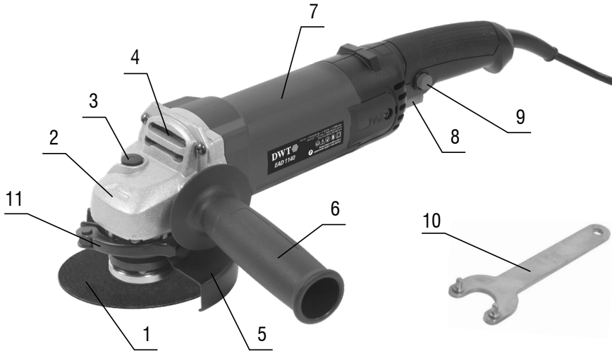
Figura 1 – Componentes da Esmerilhadeira
