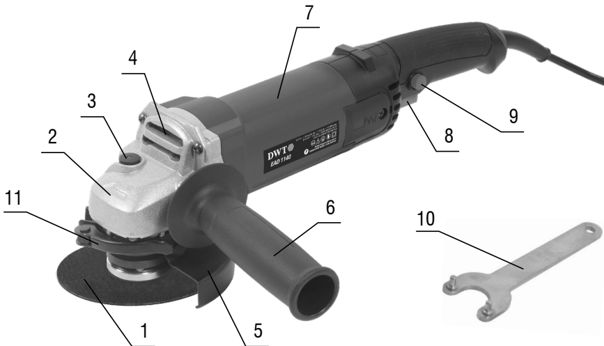
Figura 1 – Componentes de la Esmeriladora
