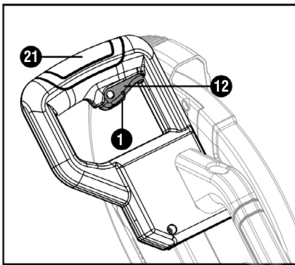
Fig. 15 – Ligando a ferramenta
