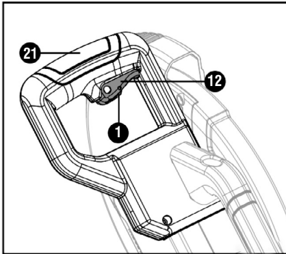
Fig. 15 – Accionamiento de la máquina
