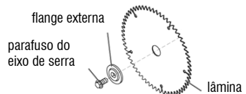
Fig. 11 – Remoção da lâmina
