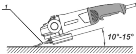
Fig. 11 – Ángulo correcto de esmerilado
