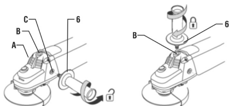
Fig. 2 – Cambio de posición del mango auxiliar
