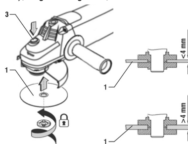
Fig. 5 – Montaje del disco en la herramienta
