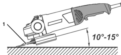
Figura 8 – Ângulo correto de esmerilhamento
