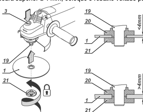
Figura 5 – Montagem do disco na máquina
