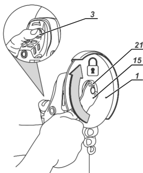
Figura 6 – Montagem do disco na máquina
