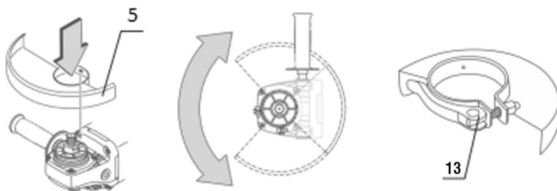
Figura 3 – Montaje y posicionamiento de la cubierta de protección
