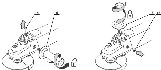
Figura 2 – Montaje de la empuñadura auxiliar
