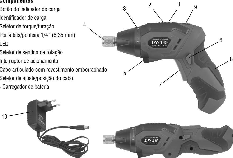
Fig. 1 – Componentes da parafusadeira PBD 360
