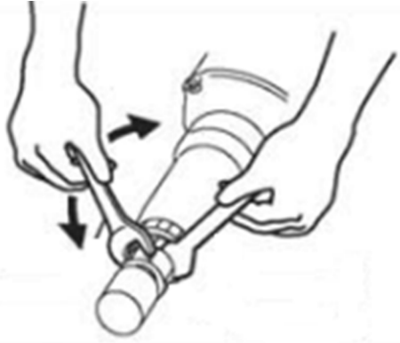
Figura 2 – Instalación de la punta montada
