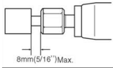
Figura 3 – Distancia entre el porta-pinza y el accesorio
