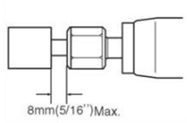
Figura 3 – Distância entre o porta-piça e o acessório
