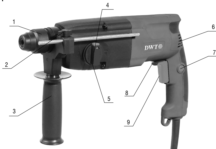
Fig. 1 – Componentes do martelete
