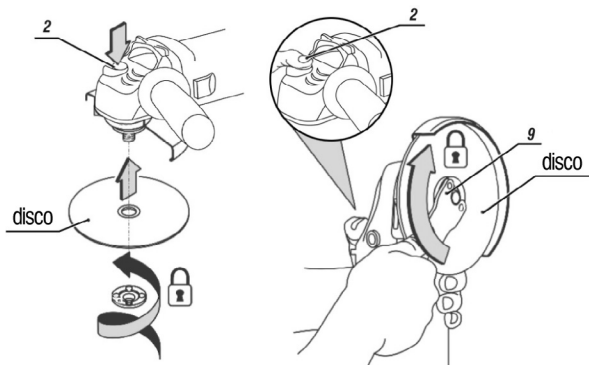
Fig. 8 – Cambiando el disco
