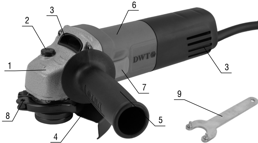
Fig. 1 – Componentes da esmerilhadeira
