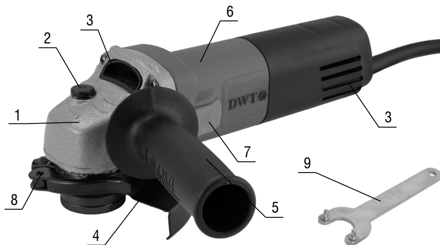
Fig. 1 – Componentes de la esmeriladora
