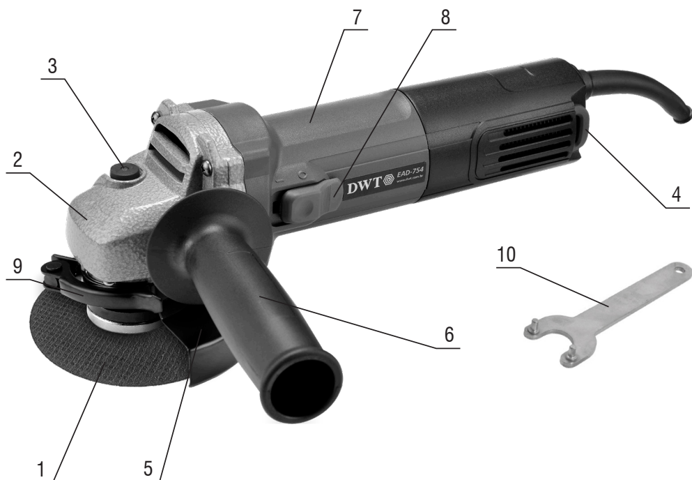
Figura 1 – Componentes de la Esmeriladora
