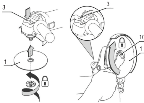
Figura 8 – Cambiando el disco
