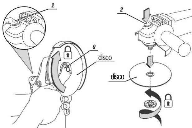
Fig. 7 – Substituição do disco
