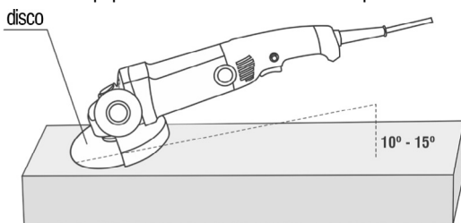
Fig. 10 – Ângulo correto de esmerilhamento
