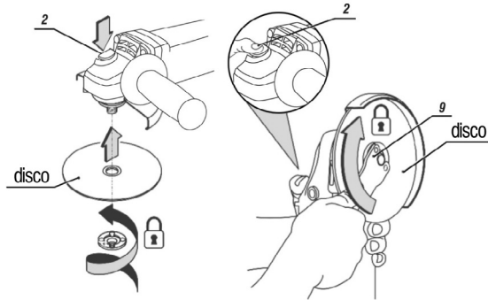
Fig. 8 – Cambiando el disco
