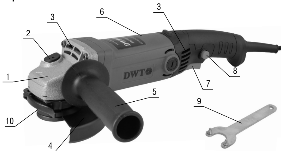
Fig. 1 – Componentes da esmerilhadeira
