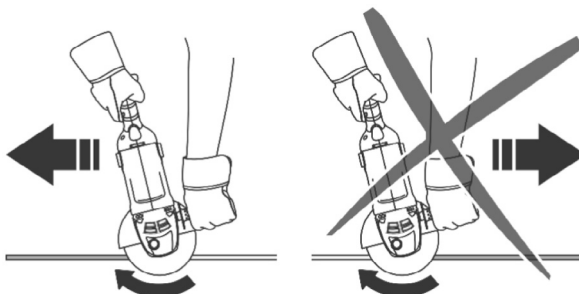
Fig. 9 – Sentido de corte correto
