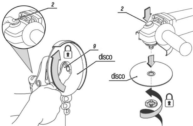
Fig. 7 – Substitución del disco
