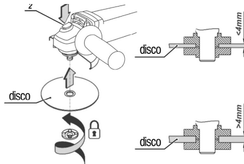
Fig. 5 – Montaje del disco en la máquina
