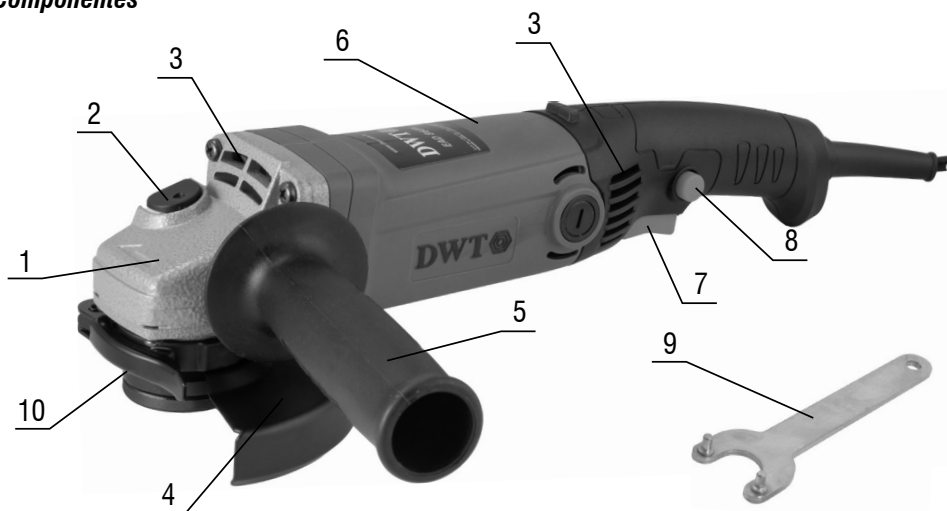
Fig. 1 – Componentes de la esmeriladora
