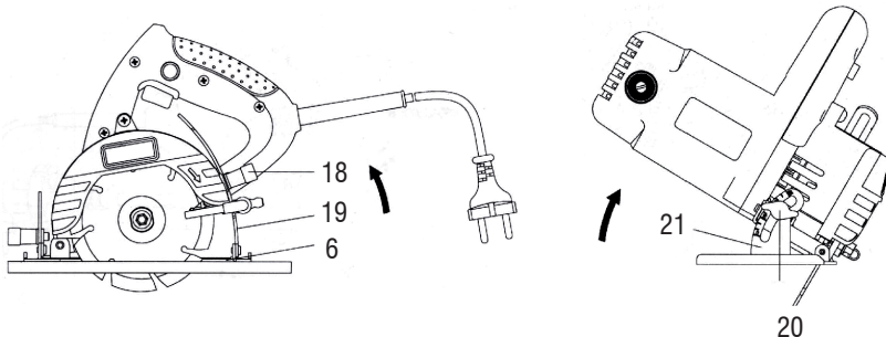
Fig. 2 - Ajuste do batente de profundidade
