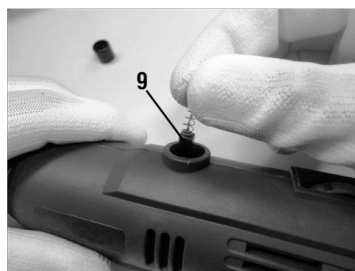
Fig. 6 – Sustitución de cepillo carbón
