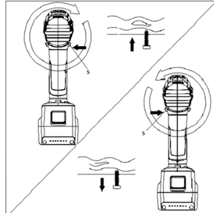
Fig. 3 – Sentido de rotación
