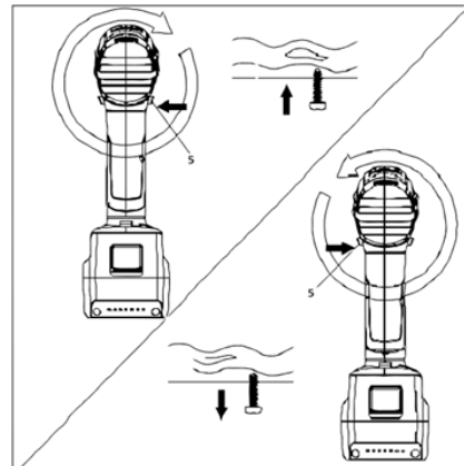
Fig. 3 – Sentido de rotação
