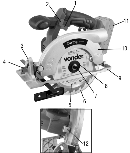
Fig. 1 – Componentes
