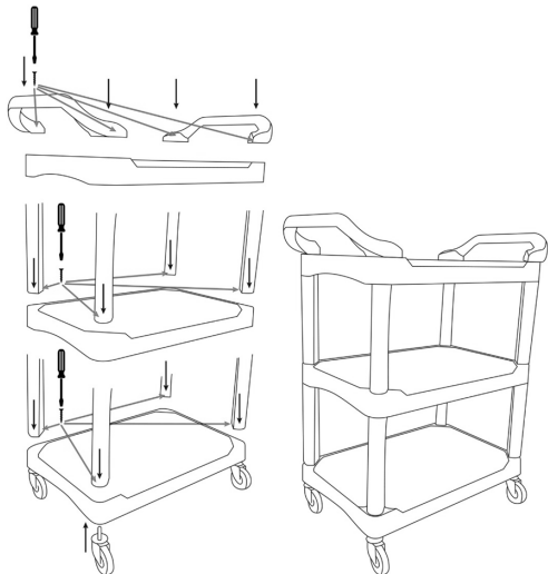
Figura 1 – Montagem do equipamento
