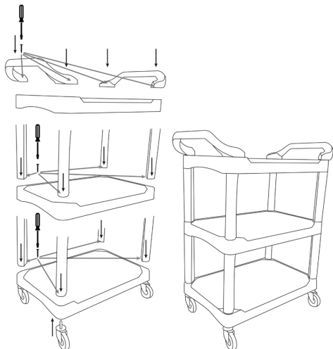
Figura 2 – Montaje del equipo
