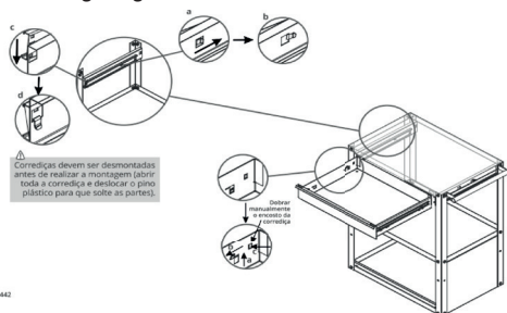
Figura 5 – Montagem da gaveta
