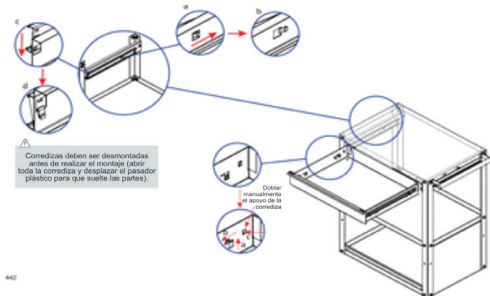
Figura 6 – Montaje cajonera
