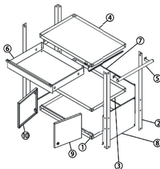
Figura 2 – Materiales
