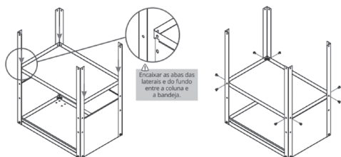
Figura 4 – Montagem bandeja intermediária
