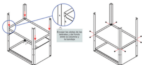
Figura 4 – Montaje bandeja intermedia
