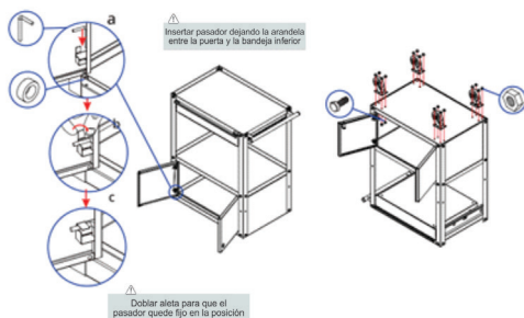
Figura 7 – Montaje puertas y ruedas
