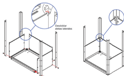
Figura 3 – Montaje bandeja inferior y laterales
