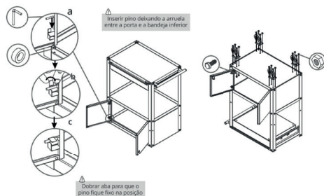
Figura 6 – Montagem portas e rodízios
