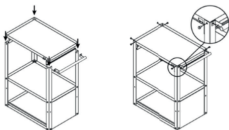
Figura 5 – Montaje bandeja superior y mango
