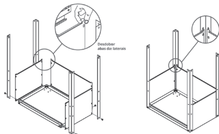
Figura 3 – Montagem bandeja inferior e laterais
