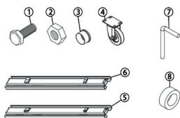
Figura 1 – Componentes
