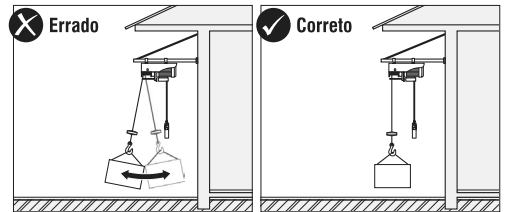
Fig. 6 – Movimiento pendular
