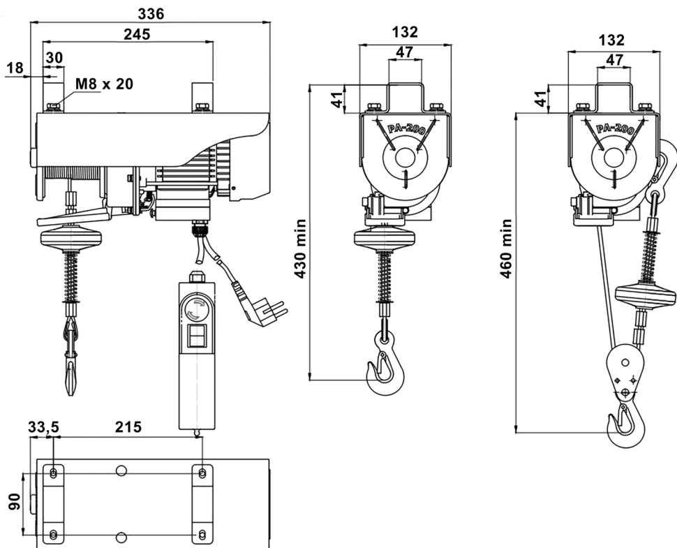
Fig. 1 – Dimensiones del producto
