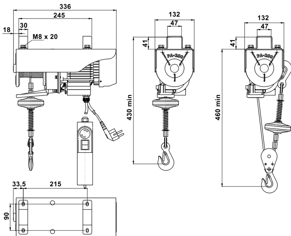
Fig. 1 – Dimensões do produto
