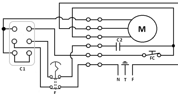
Fig. 17 – Esquema eléctrico para winche 127 V~ y 220 V~
