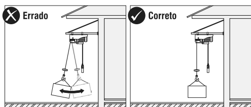
Fig. 6 – Movimento pendular
