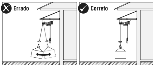
Fig. 6 – Movimiento pendular
