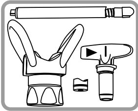
Fig. 39 – Componentes de la pistola
