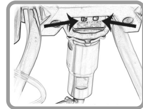
Fig. 42 – Lugar de lubricación
