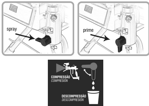
Fig. 5 – Compressão e descompressão
