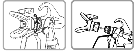
Fig. 26 – Boquilla de protección
