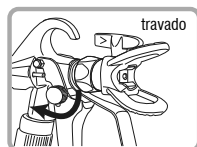
Fig. 36 – Interruptor de encendido y apagado X bloqueo del gatillo
