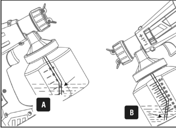
Fig. 5 – Orientación del tubo pescador
