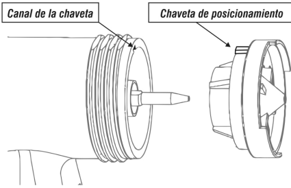
Fig. 7 – Montaje de la tapa de aire
