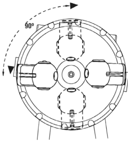
Fig. 2 – Boquilla de la pistola
