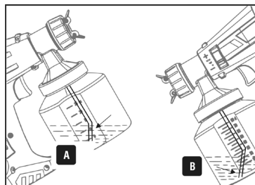
Fig. 5 – Posicionamento do tubo pescador
