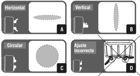
Fig. 3 – Ajuste del chorro de pintura
