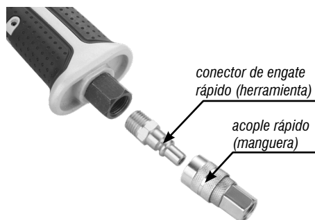
Fig. 2 – Entrada de aire
