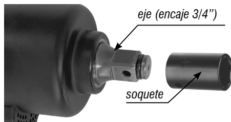
Fig. 3 – Encaje del soquete
