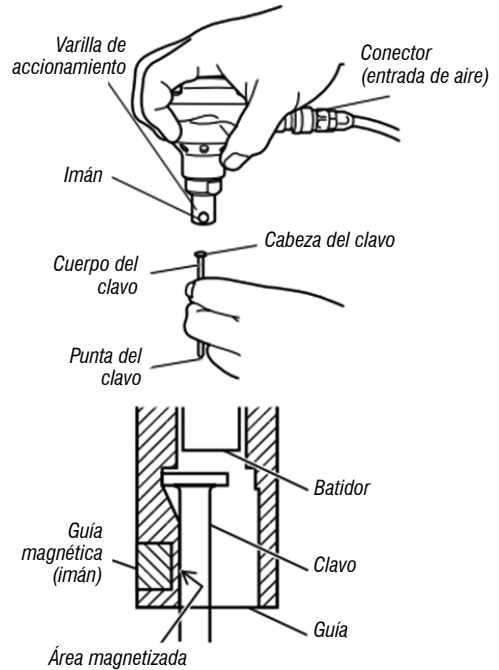
Fig. 1 – Componentes de la Mini-clavador neumático
