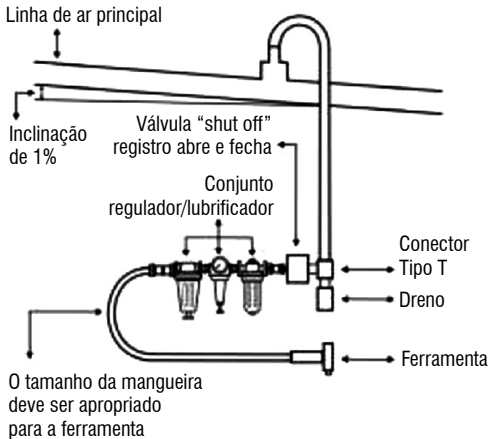
Fig. 8 – Projeto de rede de ar comprimido
