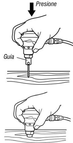
Fig. 5 – Fijación del clavo
