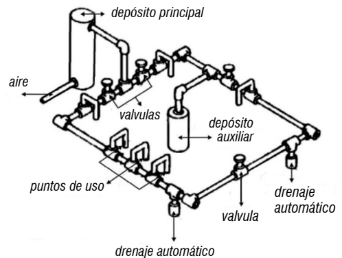
Fig. 7 – Red de aire comprimido
