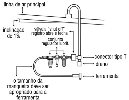
Fig. 8 – Projeto de rede de ar comprimido
