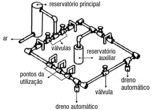
Fig. 7 – Rede de ar comprimido
