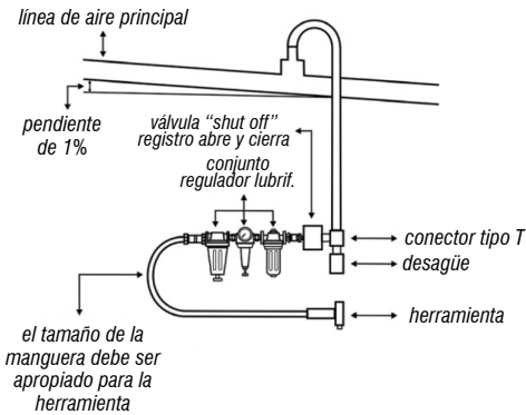
Fig. 8 – Diseño de redes de aire comprimido
