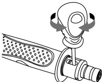
Fig. 3 – Chave para ajuste de torque
