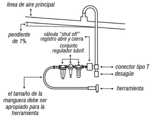
Fig. 8 – Diseño de redes de aire comprimido
