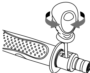
Fig. 3 – Llave de ajuste de torque
