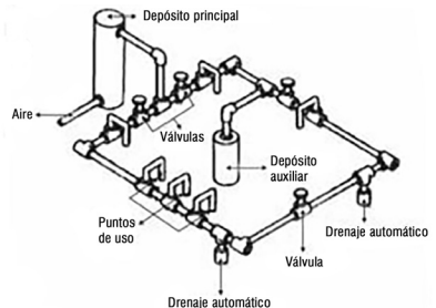
Fig. 1 – Red de aire comprimido
