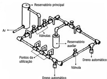
Fig. 1 – Rede de ar comprimido
