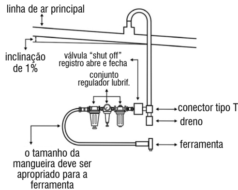
Fig. 7 – Projeto de rede de ar comprimido
