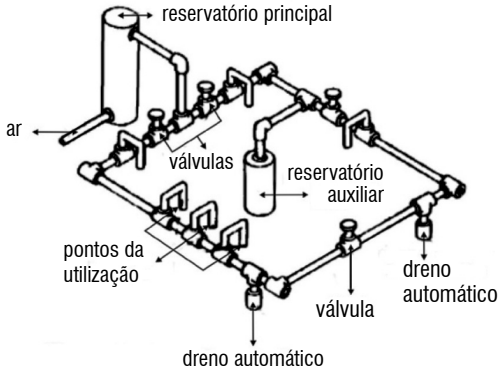
Fig. 6 – Rede de ar comprimido
