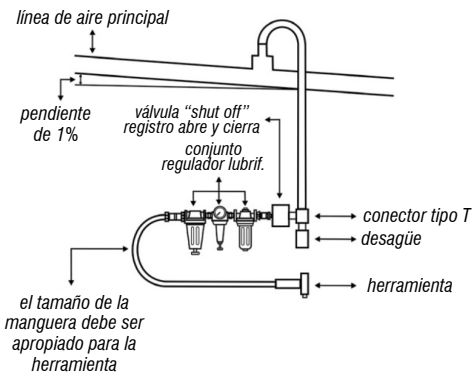
Fig. 7 – Diseño de redes de aire comprimido
