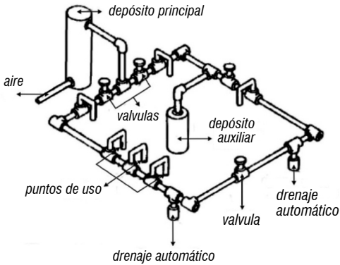
Fig. 6 – Red de aire comprimido
