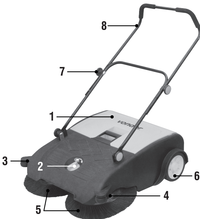
Figura 1 – Componentes da varredeira manual
