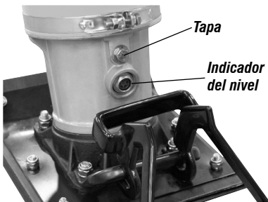
Fig. 2 – Aceite de la caja de engranajes
