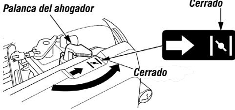
Fig. 5 – Ahogador
