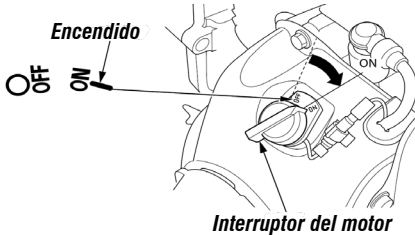
Fig. 6 – Llave general
