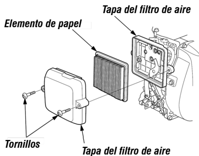
Fig. 13 – Filtro de aire
