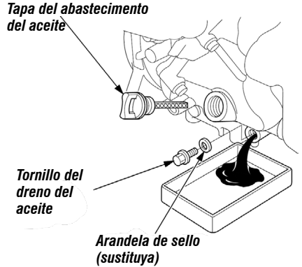
Fig. 10 – Cambio de aceite del cárter del motor
