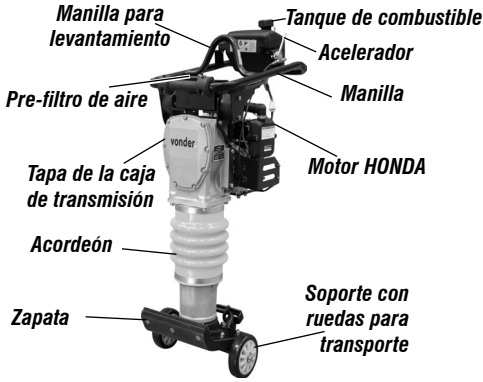
Fig. 1 – Componentes
