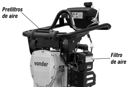
Fig. 12 – Localización de los filtros de aire
