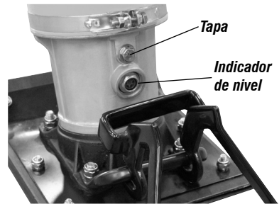
Fig. 11 – Cambio de aceite del cárter del percutor
