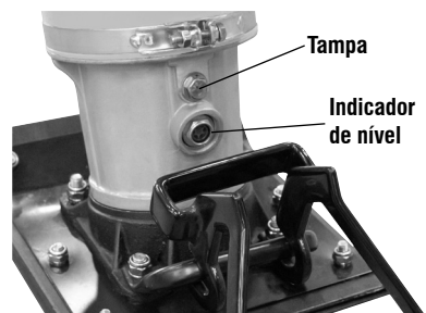
Fig. 11 – Troca de óleo do cárter do percursor
