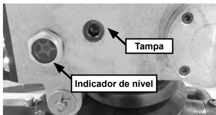
Fig. 6 – Óleo da caixa de engrenagem
