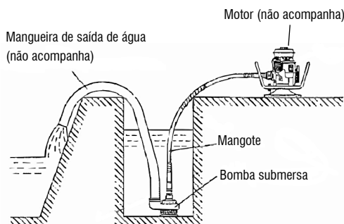
Fig. 2 – Conexão da bomba
