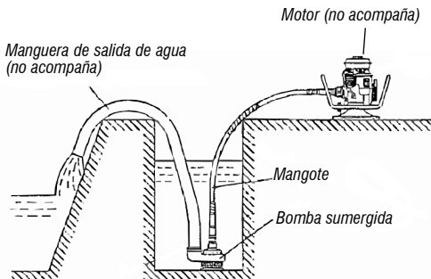
Fig. 2 – Conexión de la bomba
