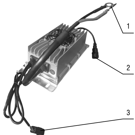
Fig. 1 – Componentes
