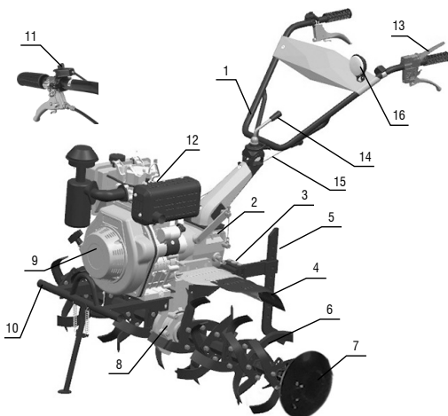
Fig. 1 – Componentes
