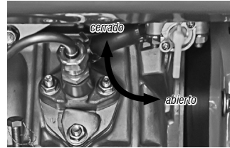
Fig. 10 – Grifo de combustible
