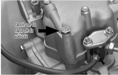
Fig. 12 – Tapón de la tapa de la válvula
