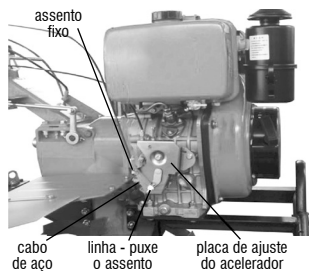
Fig. 7 – Ajuste do cabo do acelerador
