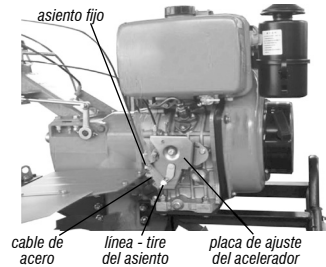
Fig. 7 - Ajuste del cable del acelerador
