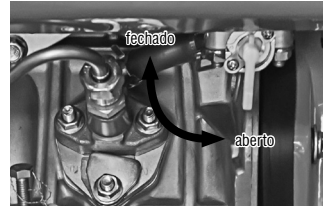
Fig. 10 – Registro de combustível
