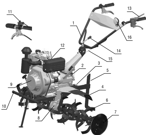
Fig. 1 – Componentes
