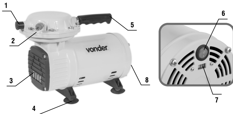
Figura 1 – Componentes do compressor
