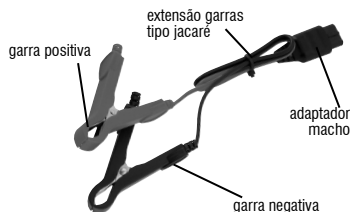
Fig. 3 – Extensão para carregamento de baterias de automóveis
