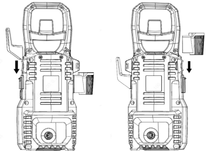
Fig. 3 – Montaje del soporte de la pistola
