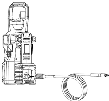
Fig. 6 – Montagem da mangueira no equipamento
