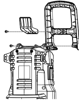
Fig. 2 – Montagem da alça de transporte
