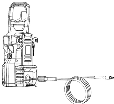
Fig. 6 – Montaje de la manguera en el equipo
