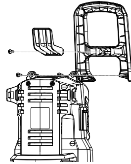
Fig. 2 – Montaje de la manilla de transporte
