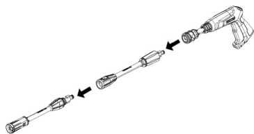
Fig. 4 – Montagem da lança
