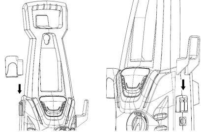
Fig. 3 – Montaje del soporte de la pistola
