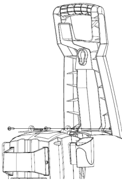
Fig. 2 – Montaje de la manilla de transporte
