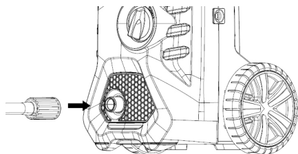
Fig. 6 – Montaje de la manguera en el equipo
