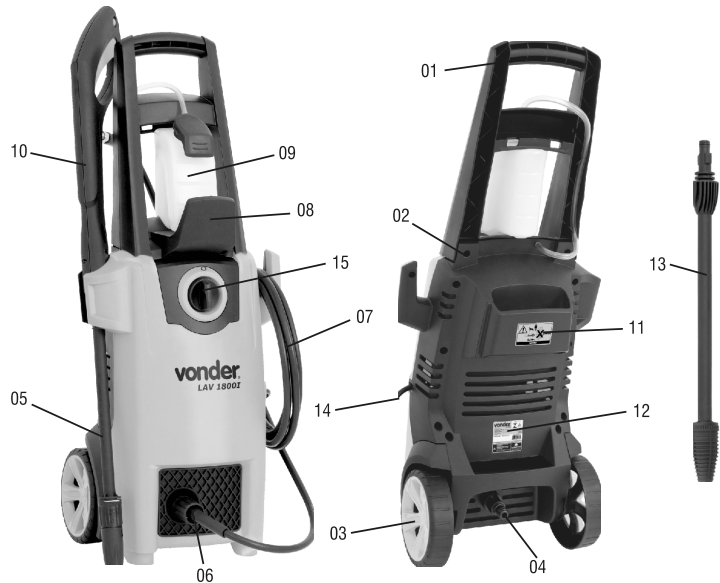
Figura 1 – Componentes de la lavadora de alta presión
