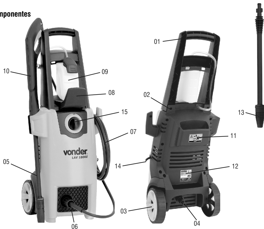
Figura 1 – Componentes da lavadora de alta pressão
