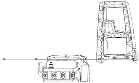
Fig. 2 – Montagem da alça de transporte
