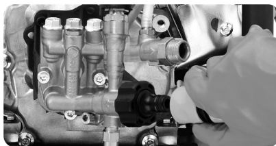
Figura 13 – Conectando a mangueira de entrada de água
