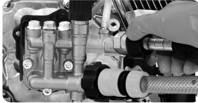
Figura 14 – Conectando la manguera de alta presión
