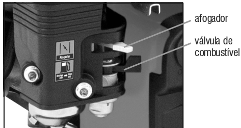
Figura 20 – Válvula de combustible y ahogador
