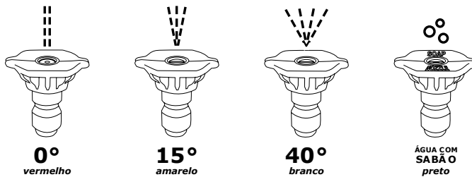
Figura 7 – Bicos de pulverização
