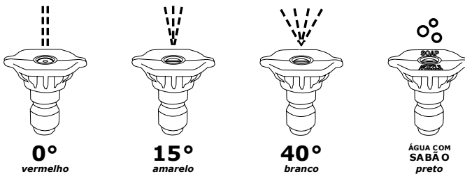
Figura 7 – Boquillas de pulverización
