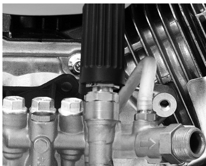
Figura 25 – Conectando la manguera de detergente en la bomba
