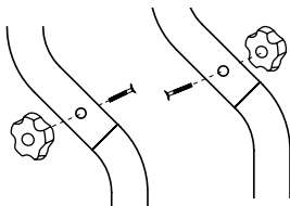
Figura 3 – Fixando a alça no suporte
