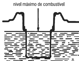
Figura 12 – Nível máximo de combustível
