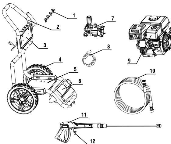
Figura 1 – Componentes da Lavadora
