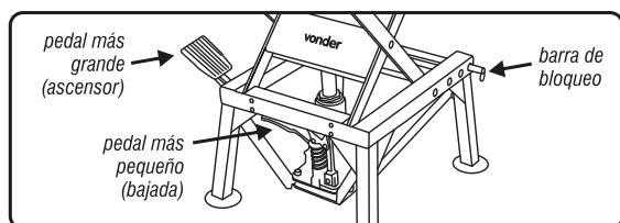
Fig. 2 - Elevación de la moto
