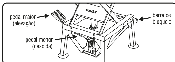
Fig. 2 - Elevação da moto
