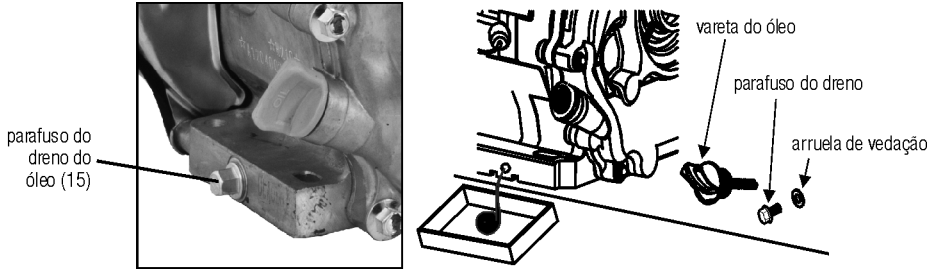
Fig. 11 – Troca de óleo
