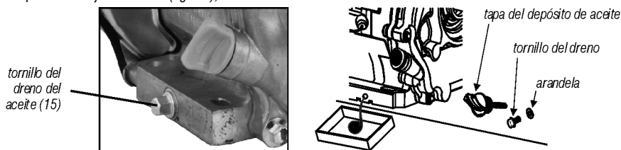
Fig. 11 - Cambio de aceite
