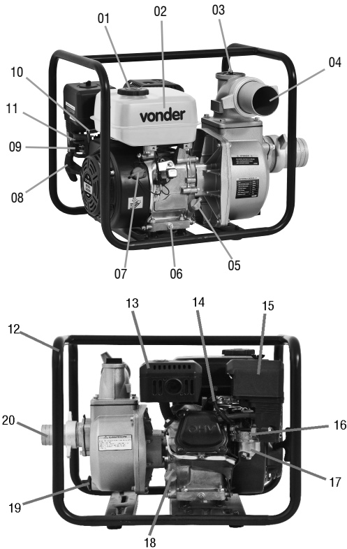
Fig. 1 – Componentes
