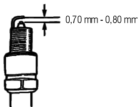
Fig. 35 – Folga da vela
