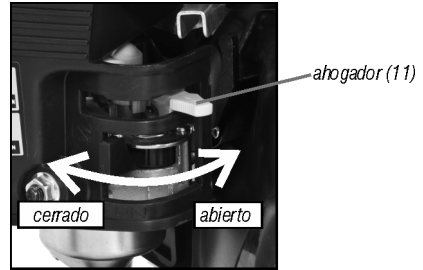
Fig. 19 – Ahogador
