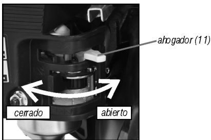
Fig. 14 – Ahogador
