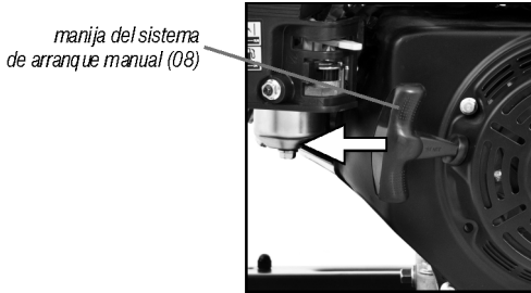
Fig. 17 – Manija del sistema de arranque
