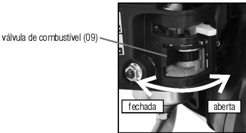
Fig. 13 – Válvula de combustível
