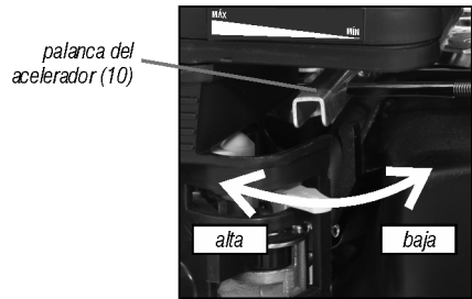
Fig. 15 – Acelarador
