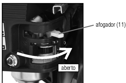
Fig. 23 – Retornando o afogador para posição aberta
