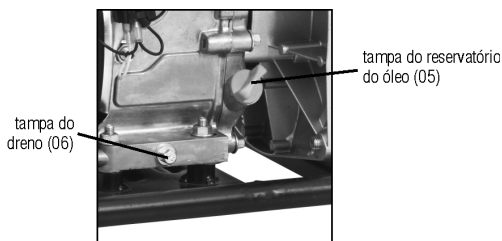
Fig. 10 – Tampa do reservatório de óleo (vareta)
