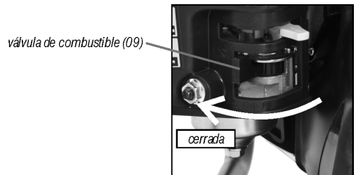
Fig. 26 – Válvula de combustible
