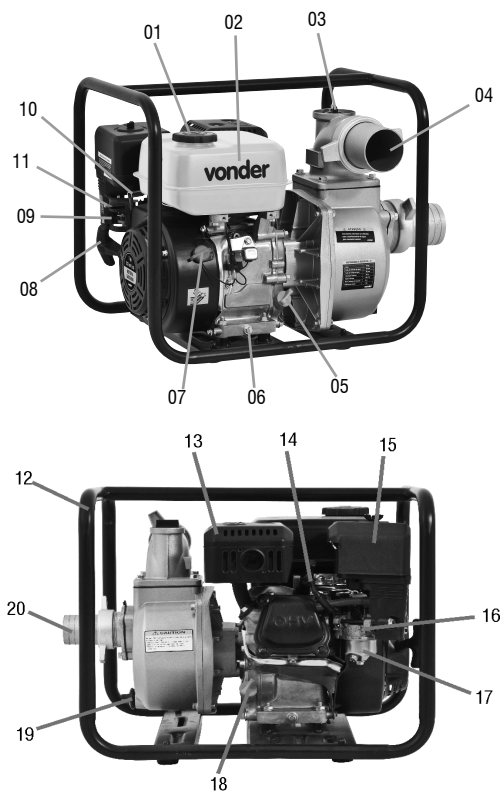
Fig. 1 – Componentes
