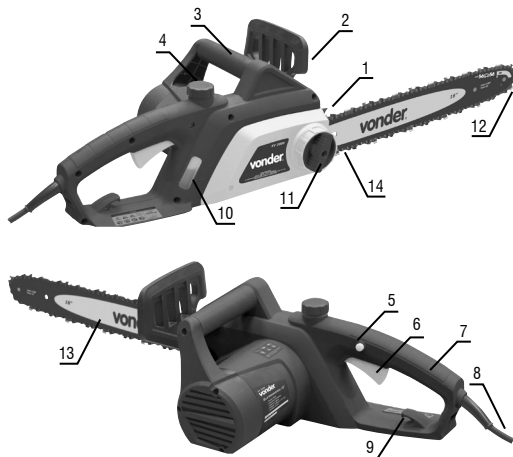
Fig. 2 – Componentes
