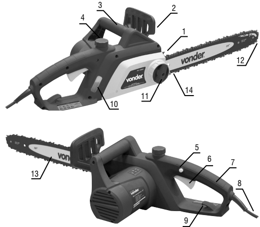
Fig. 2 – Componentes
