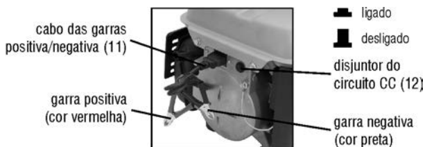
Fig. 9 – Disjuntor do circuito (CC)
