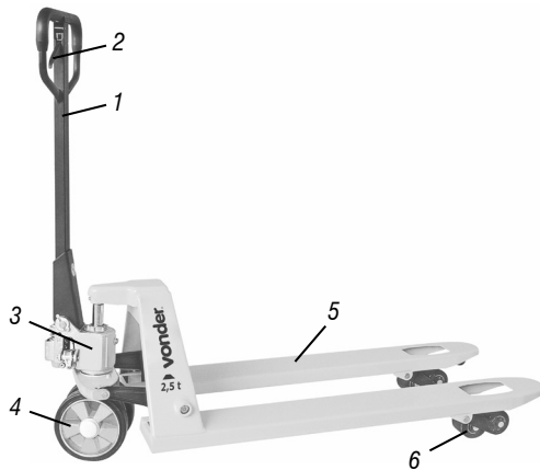
Fig. 1 – Componentes
