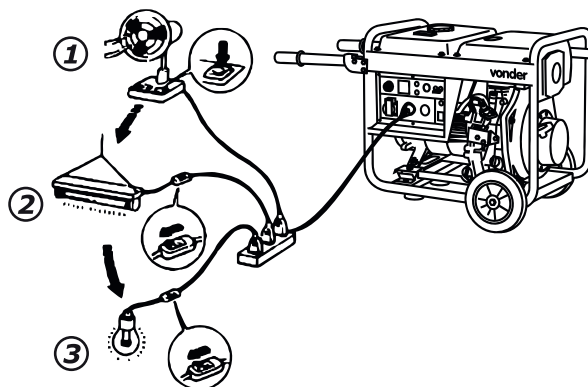
Figura 6 – Sequência de acionamento dos equipamentos
