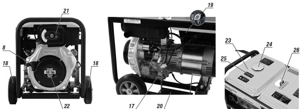
Figura 1 – Componentes do gerador
