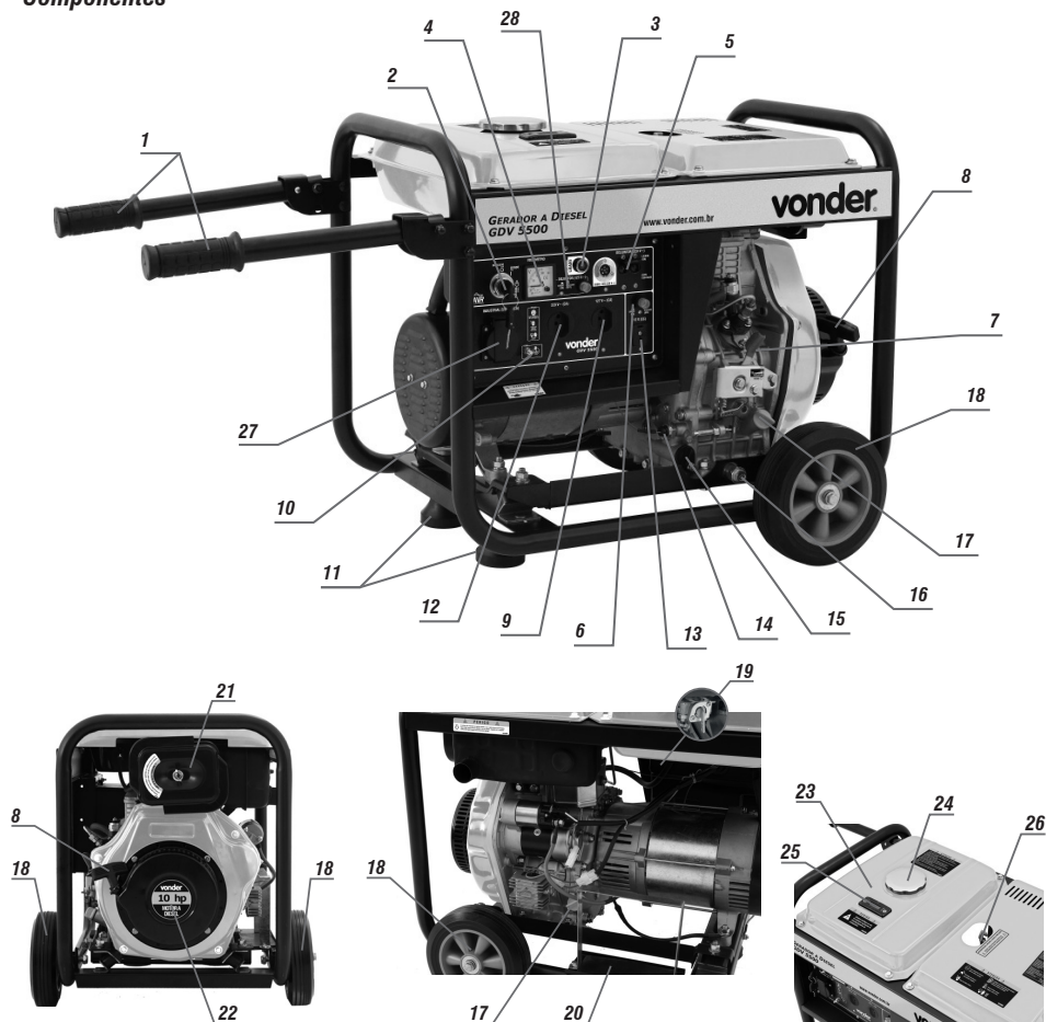
Figura 1 – Componentes del generador
