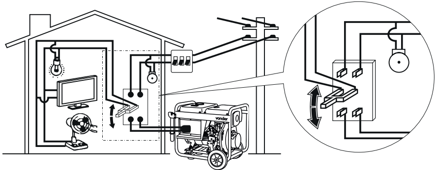
Figura 4 – Exemplo de ligação correta
