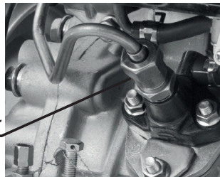
Figura 19 – Expurgando sistema de combustible
