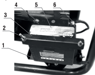
Figura 9 – Instalación de la batería
