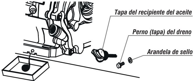
Figura 20 – Tapa del aceite (varilla)
