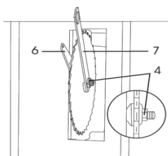
Fig. 16 – Retirando o flange do eixo para substituição da lâmina da serra
