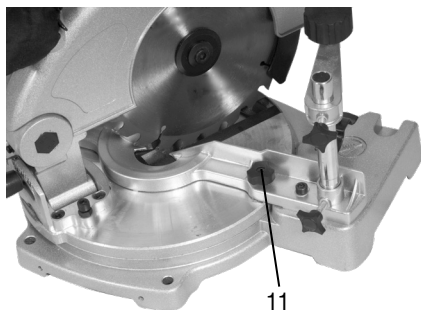
Fig. 6 – Regulagem do esquadro
