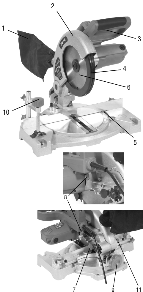
Fig. 1 – Componentes
